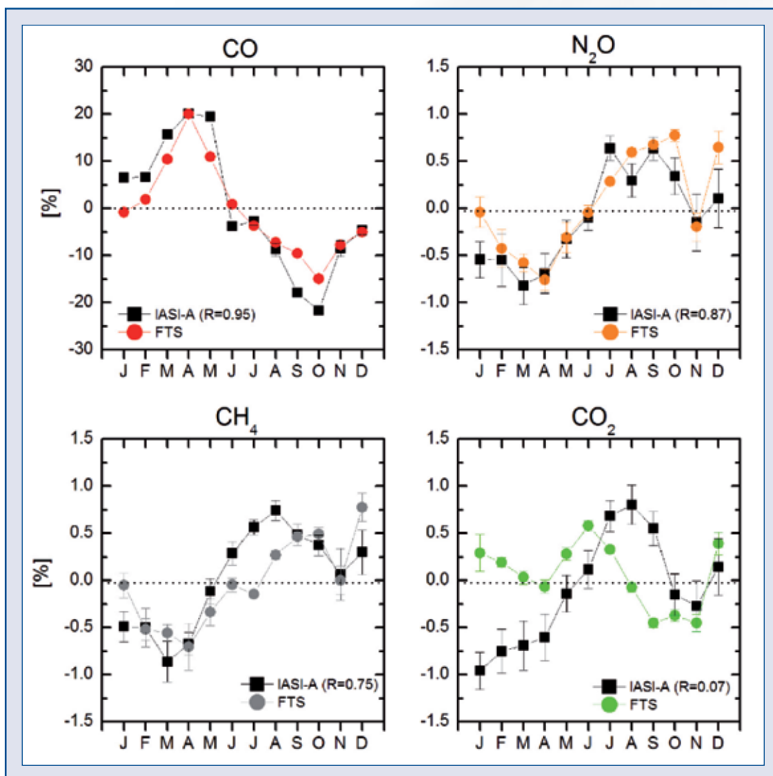
Resultados de la validación estacional del contenido de varios componentes atmosféricos (CO, N 2 O, CH 4 y CO 2 ) en la columna atmosférica medidos por IASI (EUMETSAT), utilizando como referencia las medidas de estos componentes en Izaña utilizando la técnica de espectroscopía infrarroja de Transformada de Fourier en el marco del proyecto NOVIA.
