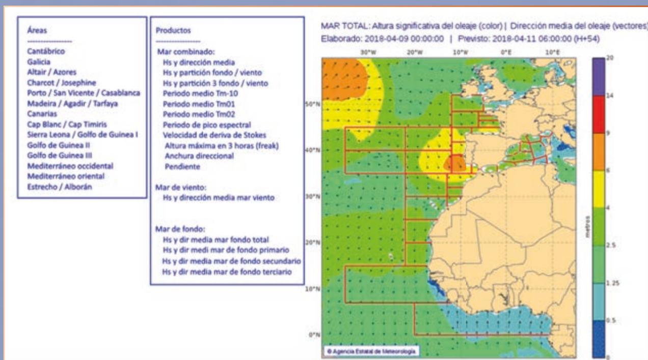
Áreas y productos. Ejemplo de producto gráfico que engloba el área de modelización: Altura significativa del mar combinado con la dirección media
