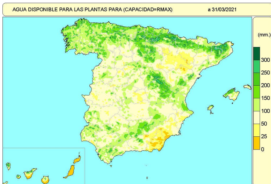
Mapa 5 Agua disponible para las plantas, o reserva de humedad edáfica en mm, considerando la capacidad de retención máxima del lugar, el día 31 de marzo de 2021.
