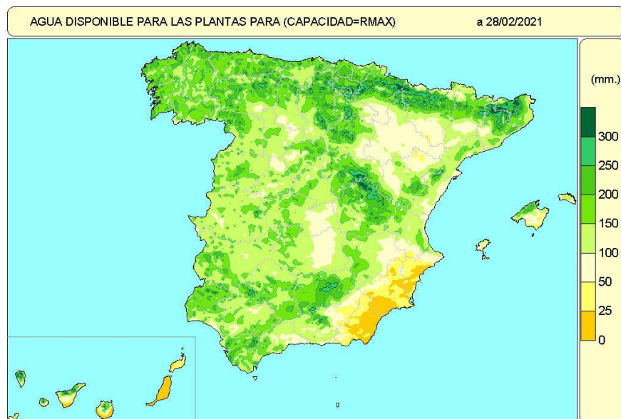
Mapa 4. Agua disponible para las plantas, o reserva de humedad edáfica en mm, considerando la capacidad de retención máxima del lugar, el día 28 de febrero de 2021.
